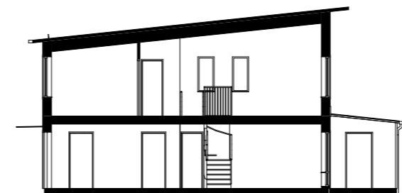
PRINCIPSEKTION
