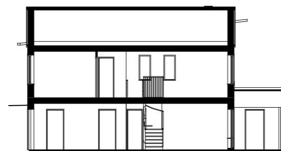
PRINCIPSEKTION
