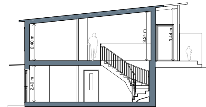
PRINCIPSEKTION
