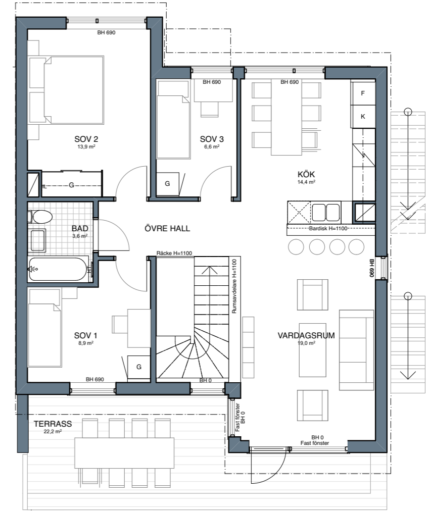
ÖVRE VÅNING
