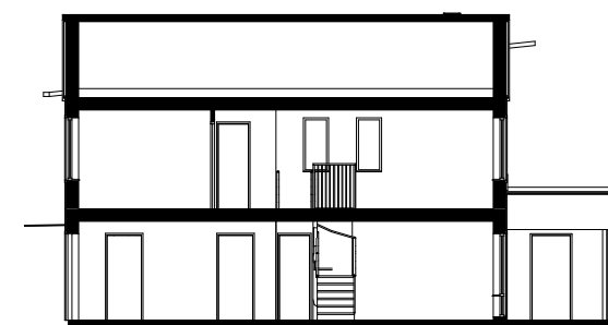
PRINCIPSEKTION
